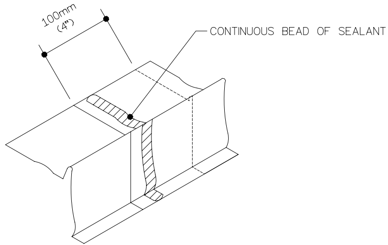
EDGE FLASHING
